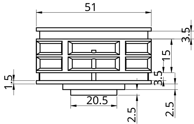
Front 1:1
